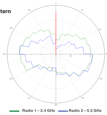
H-Plane Pattern
